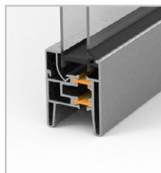
FVE S PŘERUŠENÝM TEPELNÝM MOSTEM
